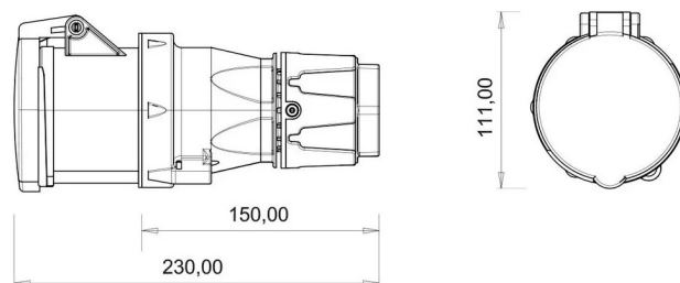
ГАБАРИТНЫЙ ЧЕРТЁЖ
