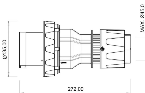
ГАБАРИТНЫЙ ЧЕРТЁЖ
