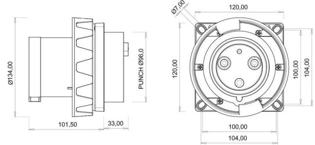
ГАБАРИТНЫЙ ЧЕРТЁЖ
