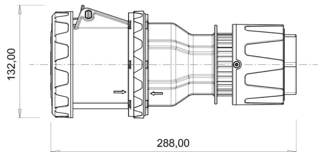
ГАБАРИТНЫЙ ЧЕРТЁЖ
