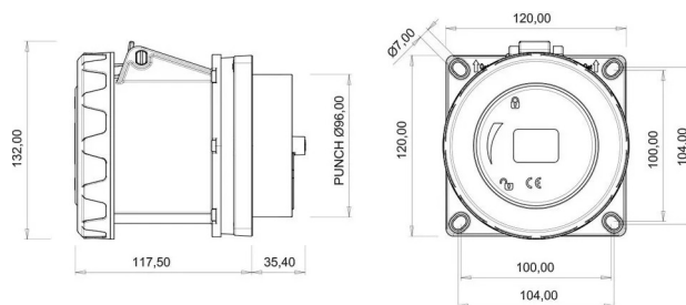
ГАБАРИТНЫЙ ЧЕРТЁЖ
