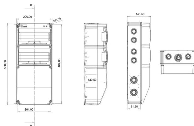
ГАБАРИТНЫЙ ЧЕРТЁЖ
