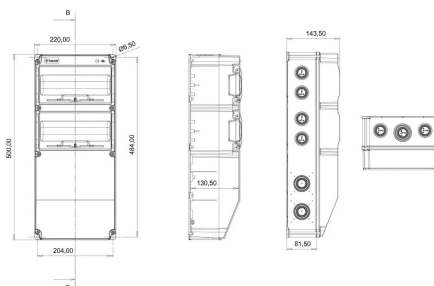
ГАБАРИТНЫЙ ЧЕРТЁЖ
