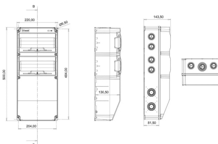
ГАБАРИТНЫЙ ЧЕРТЁЖ
