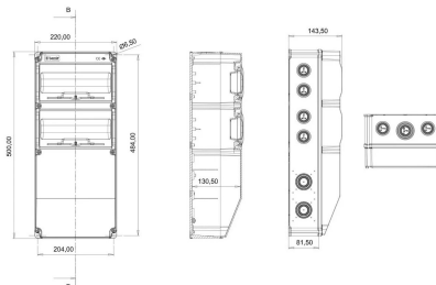
ГАБАРИТНЫЙ ЧЕРТЁЖ
