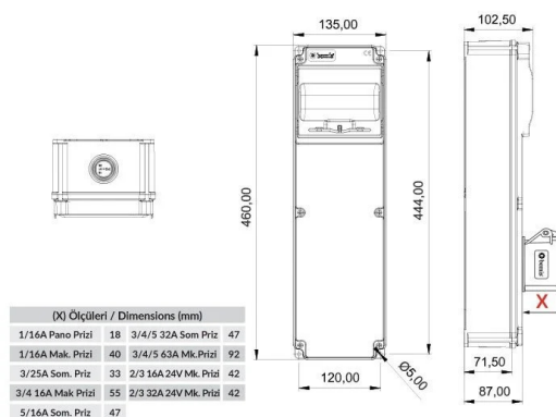
ГАБАРИТНЫЙ ЧЕРТЁЖ
