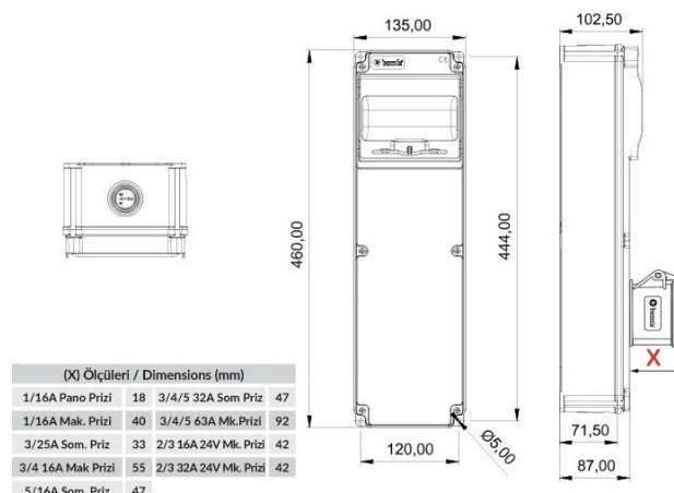
ГАБАРИТНЫЙ ЧЕРТЁЖ
