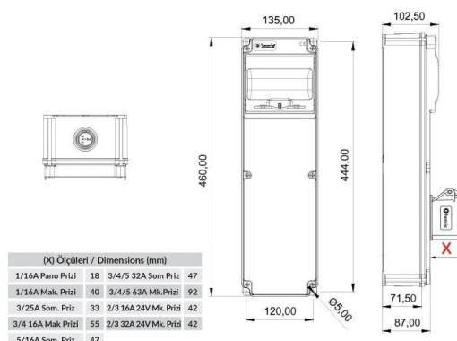
ГАБАРИТНЫЙ ЧЕРТЁЖ
