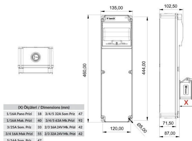
ГАБАРИТНЫЙ ЧЕРТЁЖ
