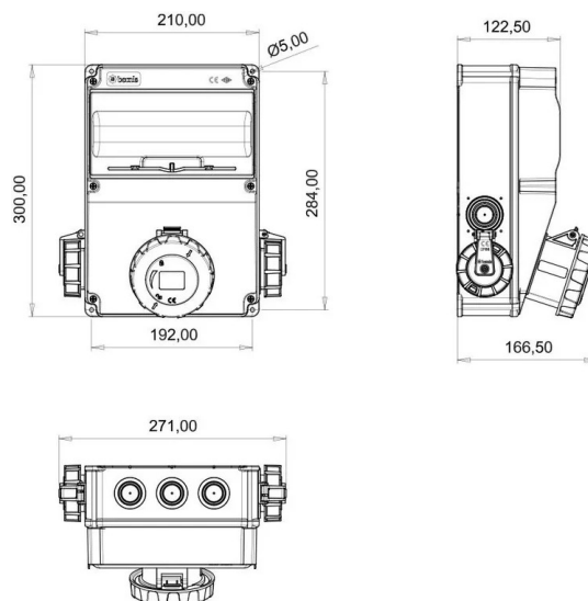
ГАБАРИТНЫЙ ЧЕРТЁЖ
