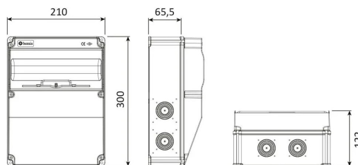
ГАБАРИТНЫЙ ЧЕРТЁЖ
