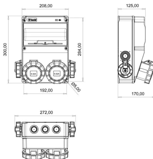
ГАБАРИТНЫЙ ЧЕРТЁЖ
