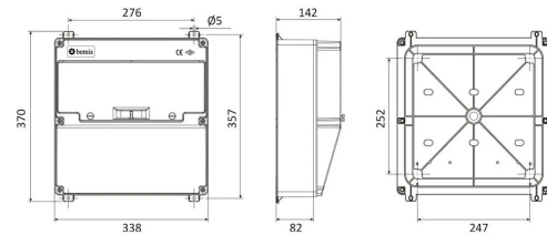
ГАБАРИТНЫЙ ЧЕРТЁЖ
