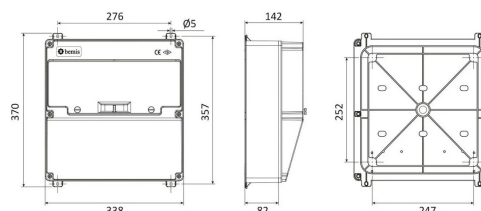
ГАБАРИТНЫЙ ЧЕРТЁЖ
