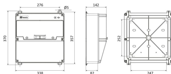
ГАБАРИТНЫЙ ЧЕРТЁЖ
