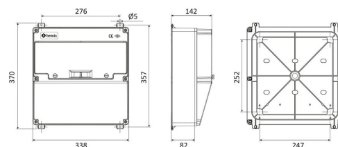
ГАБАРИТНЫЙ ЧЕРТЁЖ
