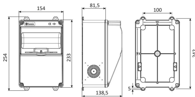
ГАБАРИТНЫЙ ЧЕРТЁЖ
