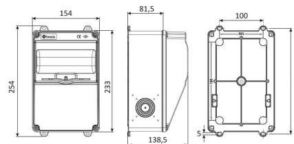
ГАБАРИТНЫЙ ЧЕРТЁЖ
