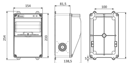
ГАБАРИТНЫЙ ЧЕРТЁЖ
