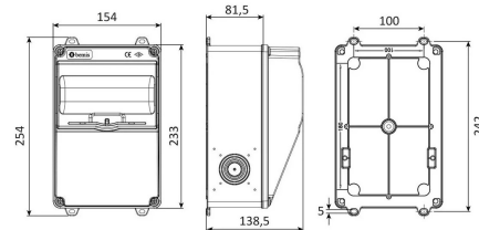
ГАБАРИТНЫЙ ЧЕРТЁЖ
