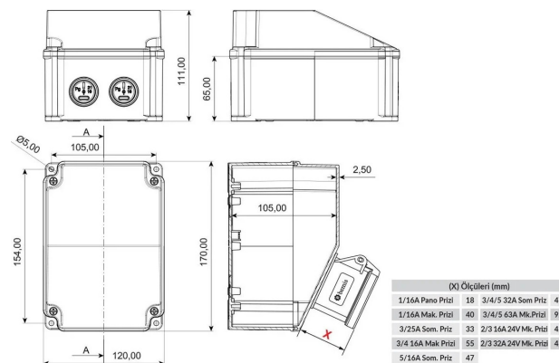
ГАБАРИТНЫЙ ЧЕРТЁЖ
