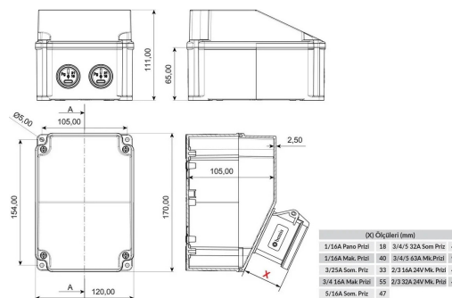
ГАБАРИТНЫЙ ЧЕРТЁЖ
