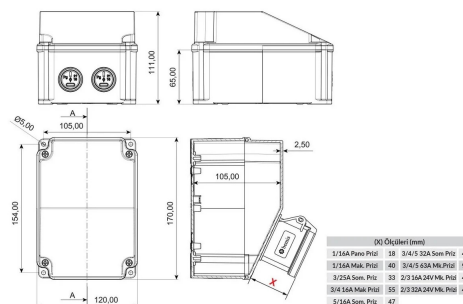
ГАБАРИТНЫЙ ЧЕРТЁЖ
