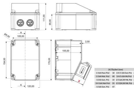
ГАБАРИТНЫЙ ЧЕРТЁЖ
