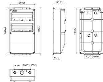
ГАБАРИТНЫЙ ЧЕРТЁЖ
