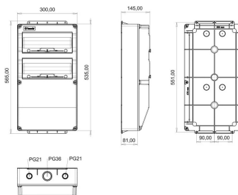
ГАБАРИТНЫЙ ЧЕРТЁЖ
