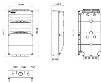
ГАБАРИТНЫЙ ЧЕРТЁЖ
