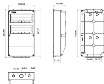
ГАБАРИТНЫЙ ЧЕРТЁЖ
