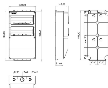
ГАБАРИТНЫЙ ЧЕРТЁЖ
