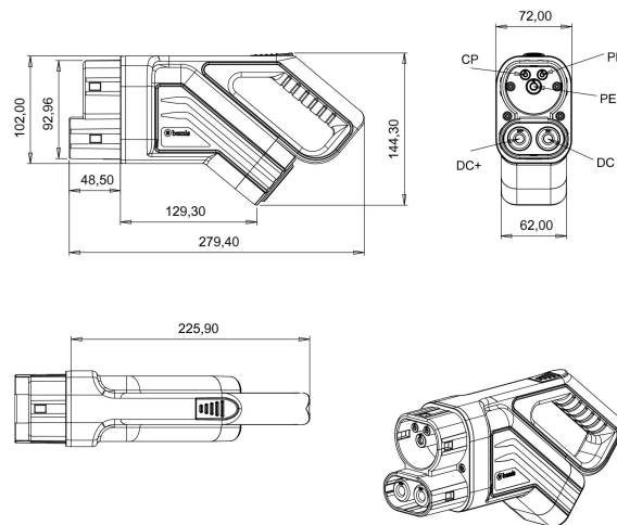
ГАБАРИТНЫЙ ЧЕРТЁЖ
