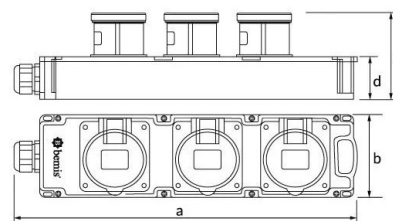
Ölçüler / Dimensions (mm)
