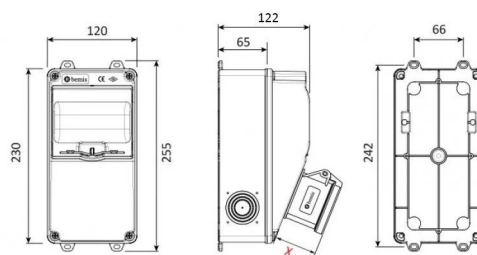
ГАБАРИТНЫЙ ЧЕРТЁЖ
