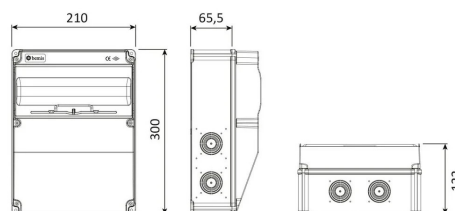
ГАБАРИТНЫЙ ЧЕРТЁЖ
