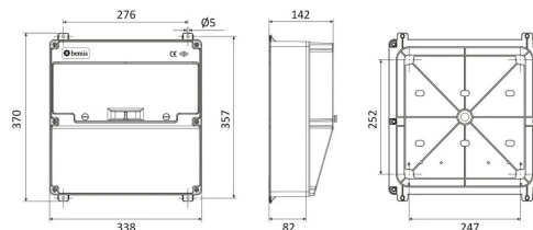
ГАБАРИТНЫЙ ЧЕРТЁЖ
