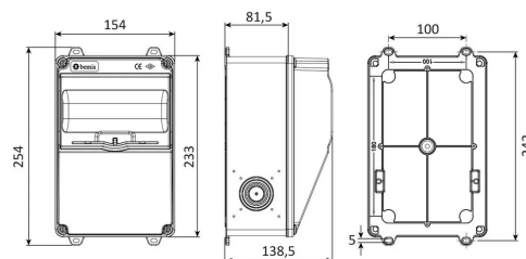
ГАБАРИТНЫЙ ЧЕРТЁЖ
