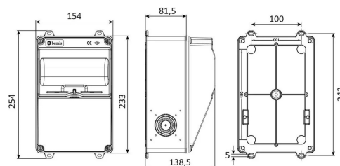
ГАБАРИТНЫЙ ЧЕРТЁЖ
