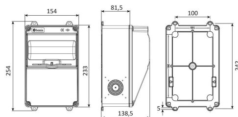
ГАБАРИТНЫЙ ЧЕРТЁЖ
