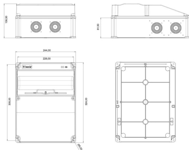
ГАБАРИТНЫЙ ЧЕРТЁЖ
