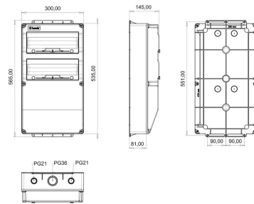
ГАБАРИТНЫЙ ЧЕРТЁЖ
