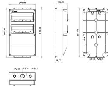
ГАБАРИТНЫЙ ЧЕРТЁЖ
