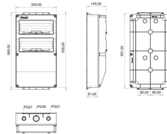
ГАБАРИТНЫЙ ЧЕРТЁЖ
