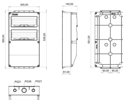
ГАБАРИТНЫЙ ЧЕРТЁЖ
