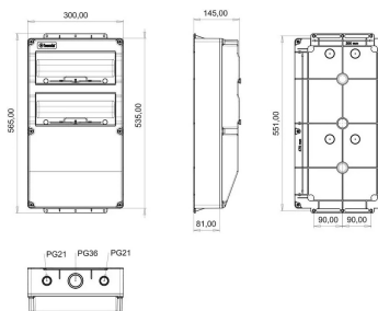
ГАБАРИТНЫЙ ЧЕРТЁЖ
