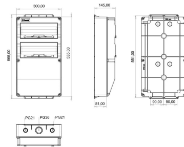
ГАБАРИТНЫЙ ЧЕРТЁЖ
