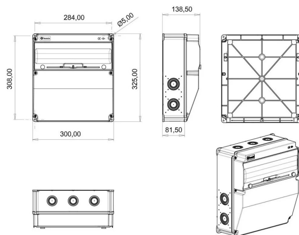
ГАБАРИТНЫЙ ЧЕРТЁЖ
