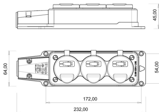
ГАБАРИТНЫЙ ЧЕРТЁЖ
